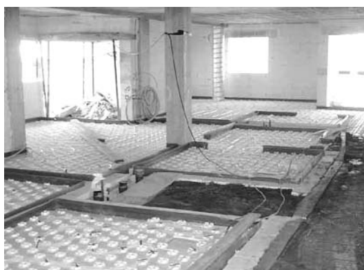
System for distribusjon av gulvvarme
